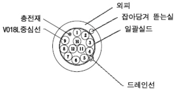
그림1. 구조도
