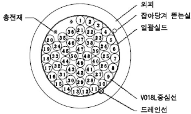
그림1. 구조도
