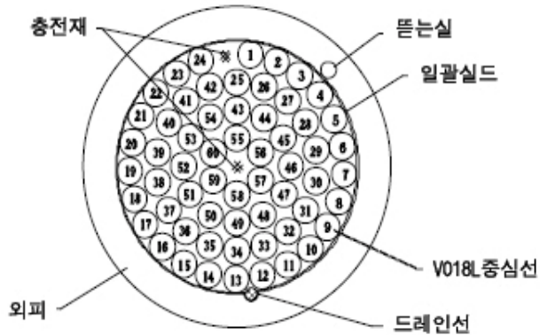
그림1. 구조도
