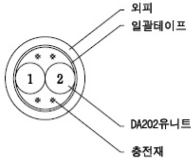
그림1. 구조도
