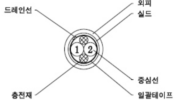
그림2. DA202 유니트구조도
