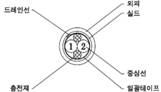
그림2. DA202 유닛구조도
