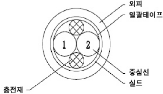
그림1. 구조도
