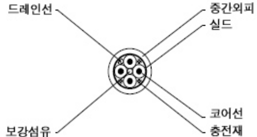
그림2. 4E3-AT-EM유니트 구조도
