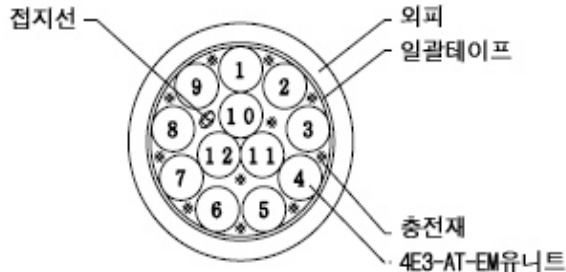
그림1. 구조도
