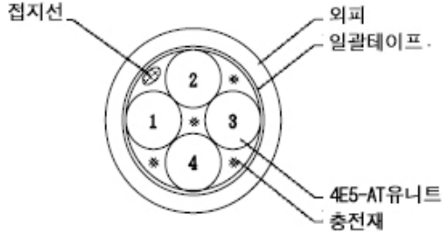
그림1. 구조도
