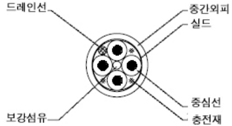
그림2. 4E5-AT유니트 구조도
