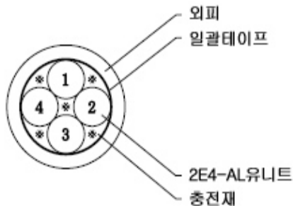
그림1. 구조도
