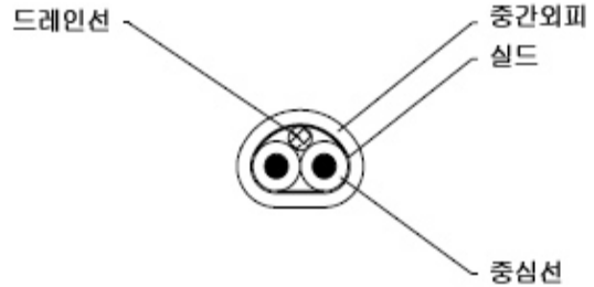
그림2. 2E4-AL유니트 구조도
