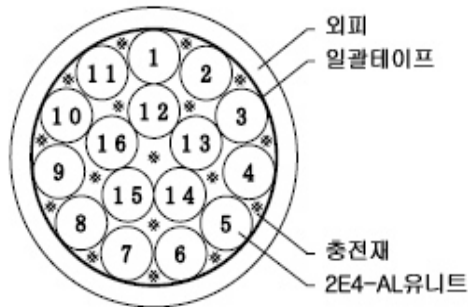
그림1. 구조도
