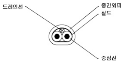
그림2. 2E4-AL유닛 구조도
