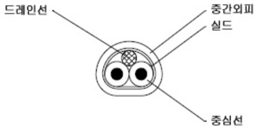
그림2. M202-AT유니트 구조도
