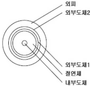
구 조 도
