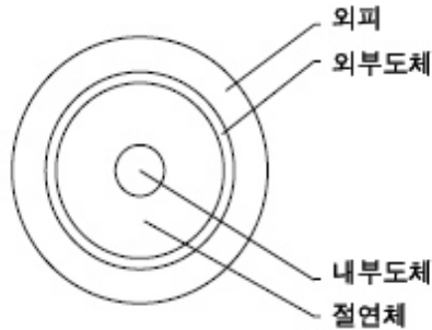
구조도
