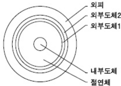
구조도
