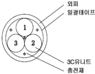
그림1. 구조도
