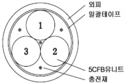
그림1. 구조도
