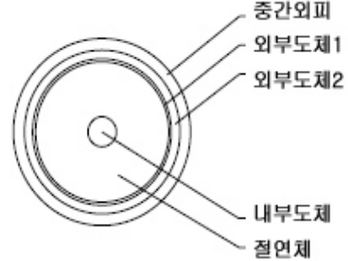
그림2. 5CFB유니트구조도
