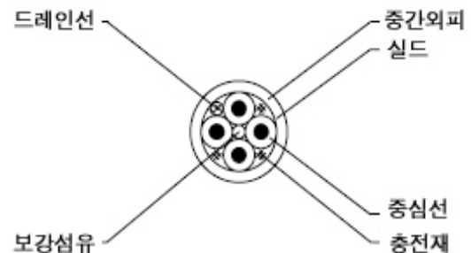
그림2. 4E4-ATG유니트 구조도
