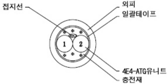
그림1. 구조도
