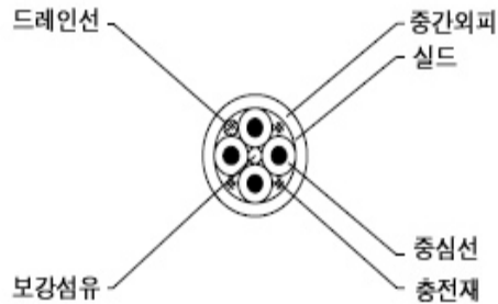
그림2. 4E4-ATG유니트 구조도
