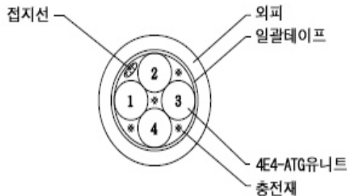
그림1. 구조도
