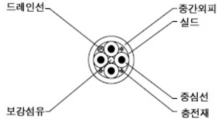
그림2. 4E4-ATG유닛 구조도
