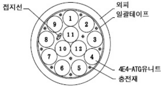
그림1. 구조도
