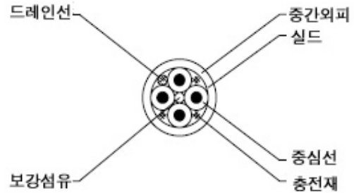
그림2. 4E4-ATG유닛 구조도
